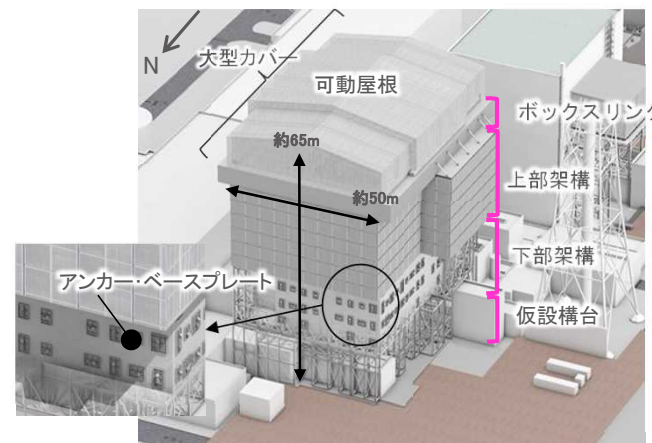
<大型カバー全体の概要図>
